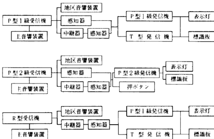
図10の2-1 無線式自動火災報知設備の構成図例
