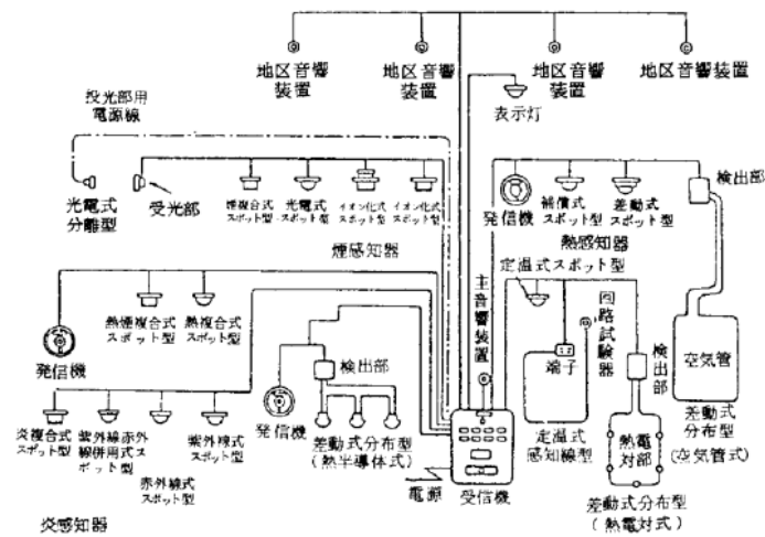
図10—1 自動火災報知設備の構成図例
